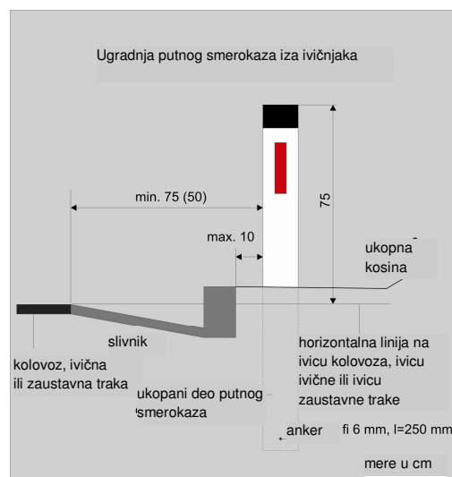
Slika 2.7.2: Putni smerokaz ugrađen uz ivičnjak
